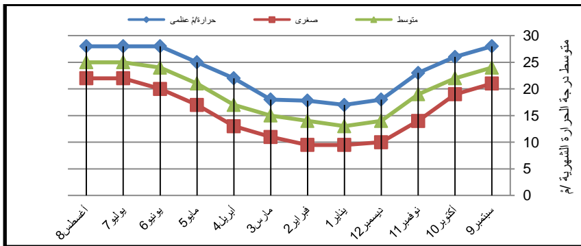
شكل (2) المتوسط الشهري لدرجات الحرارة العظمى والصغرى والمدى/م بمحطة ارضاء طريق.
